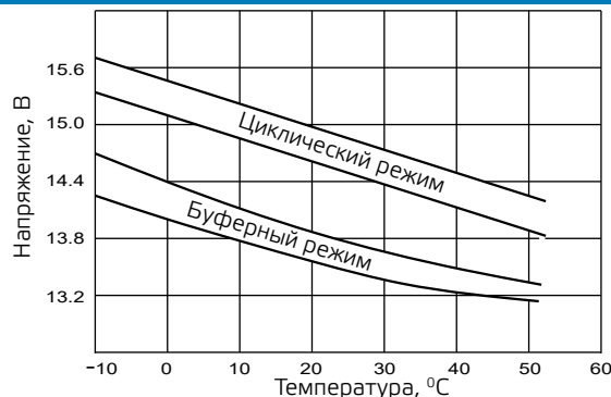
Зависимость напряжения заряда от температуры
