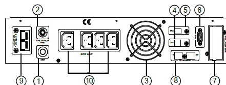
ИБП Pro OnLine 1000
