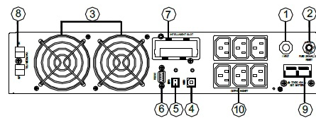
ИБП Pro OnLine 2000 и ИБП Pro OnLine 3000
