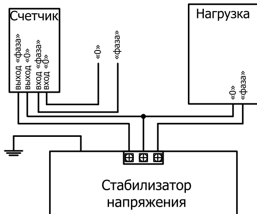
Рекомендуемая схема подключения стабилизатора к сети
